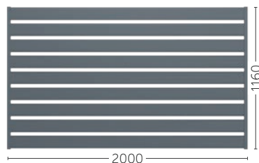
Wersja 100 9 paneli w przęśle
