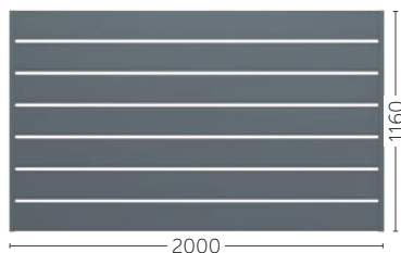
Wersja 150 7 paneli w przęśle
