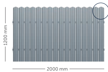
Wersja 05 Montaż pionowy 16 paneli w prześle
