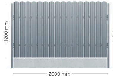
Wersja 05 PACZKA Z TWOIM OGRODZENIEM
